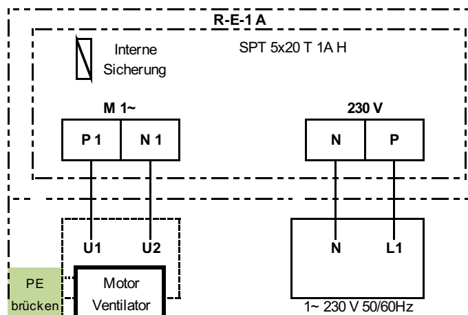
Anschlussschema
